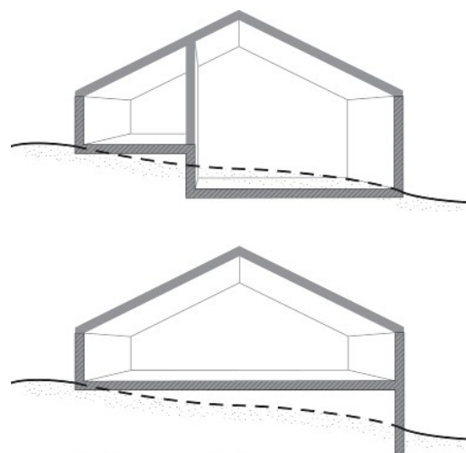
Fig. 1. Bebyggelsen skal tilpasses det eksisterende terræn. Øverst er vist bebyggelse i forskudt plan. Nederst, er vist terrænavvikling over sokkel.
